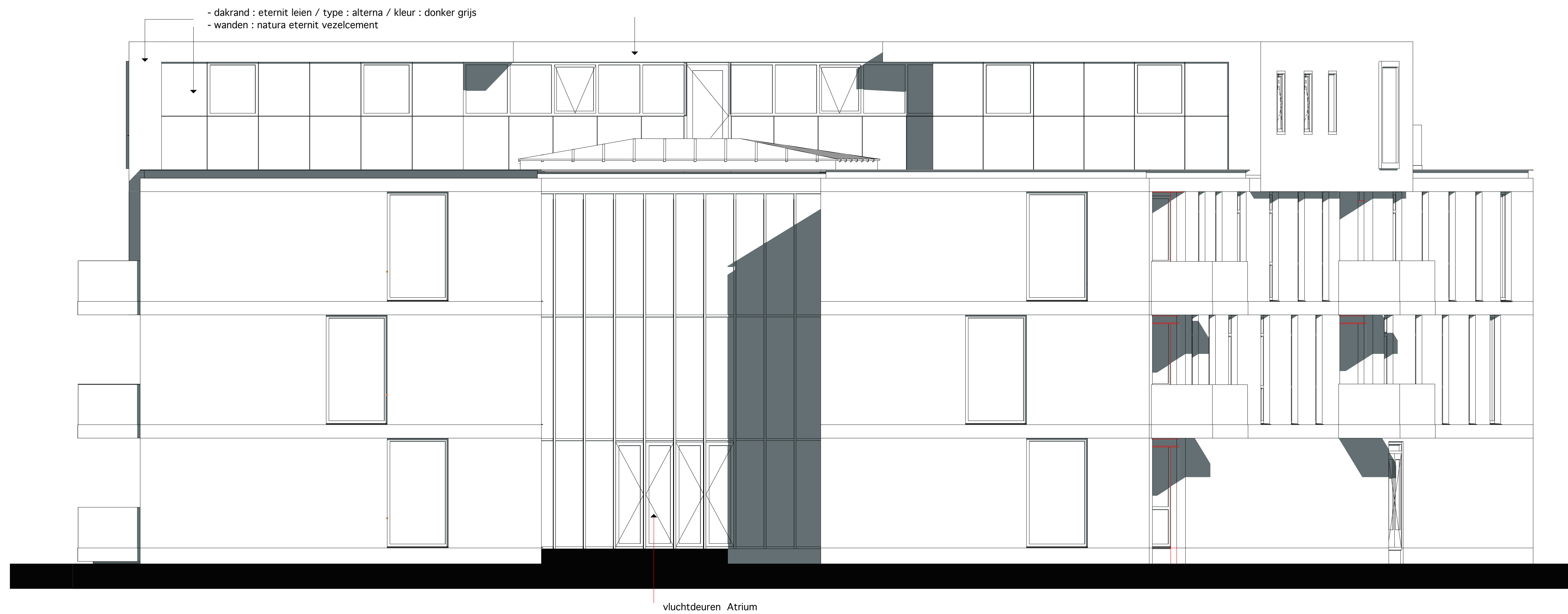
Noordgevel
